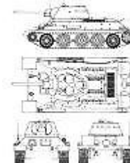
T-34-76 Modelo 1943 Perfil
